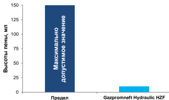
Минимизация пенообразования**
